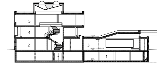
חתך של המבנה
